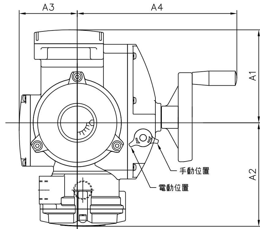
寸法表
