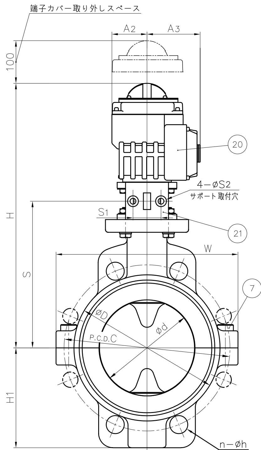
寸法表
