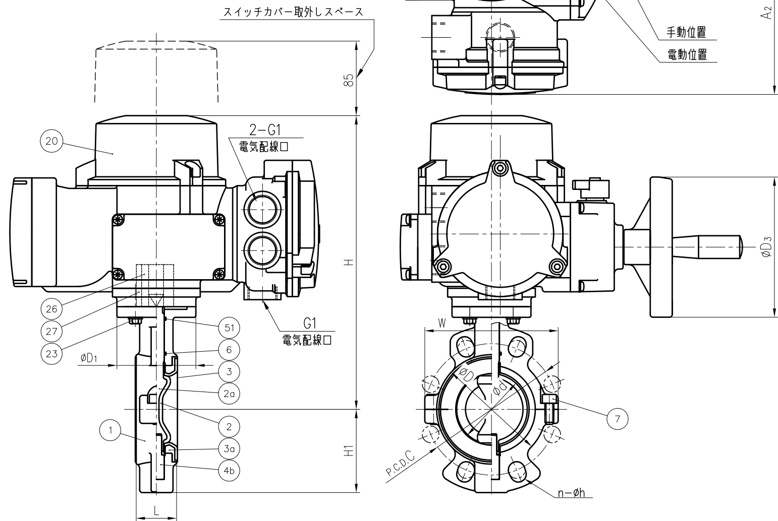
寸法表
