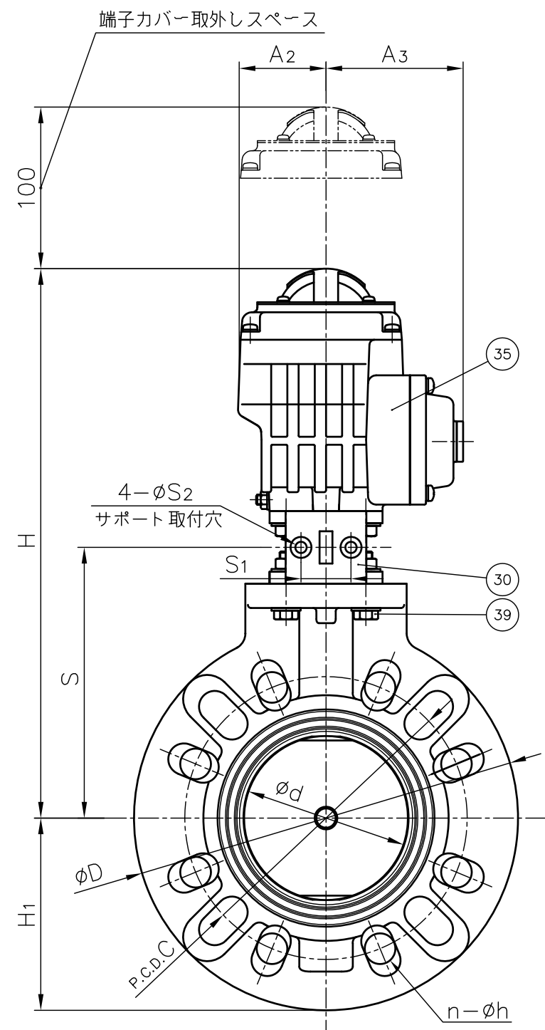
寸法表
