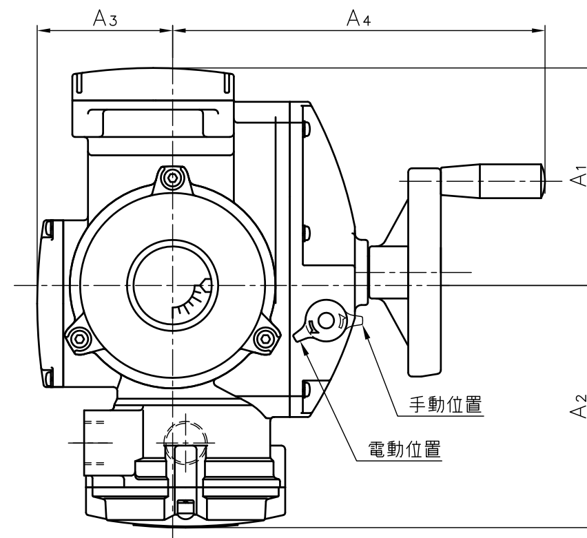
X-X矢視図
