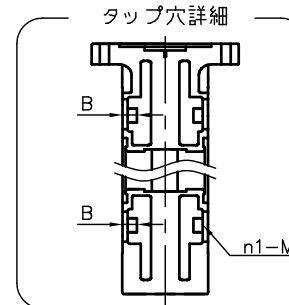
タップ穴詳細
