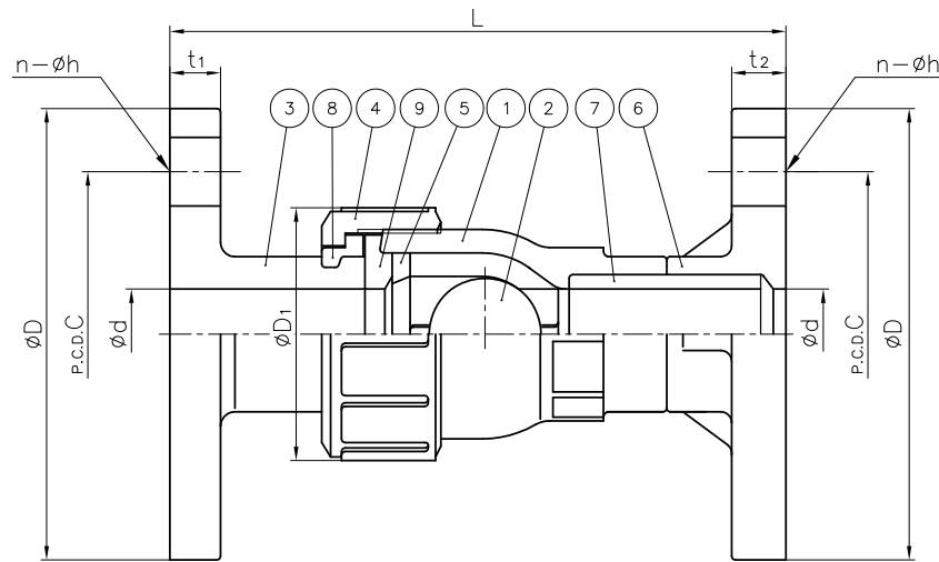
フランジ形
