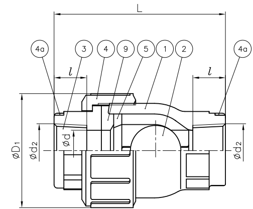
ねじ込み形
