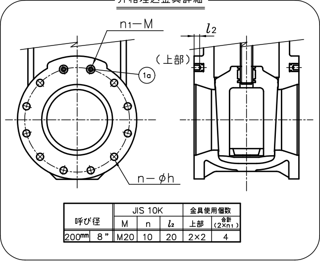
弁箱埋込金具詳細
