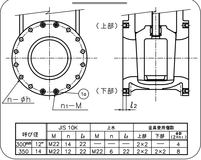
弁箱埋込金具詳細
