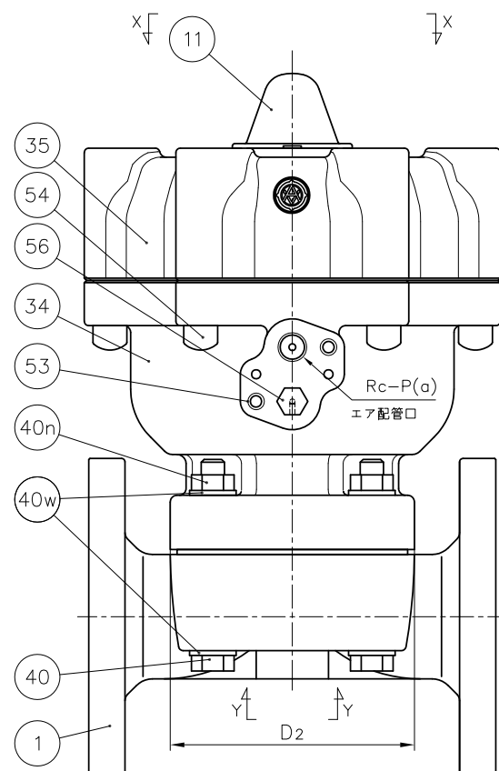
ダイヤフラムがPTFEの場合
