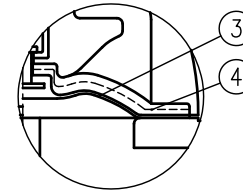
ダイアフラム材質がPTFEの場合
