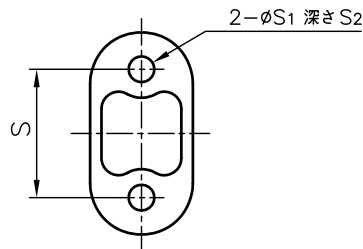
(エンザート金具取付穴部詳細)
