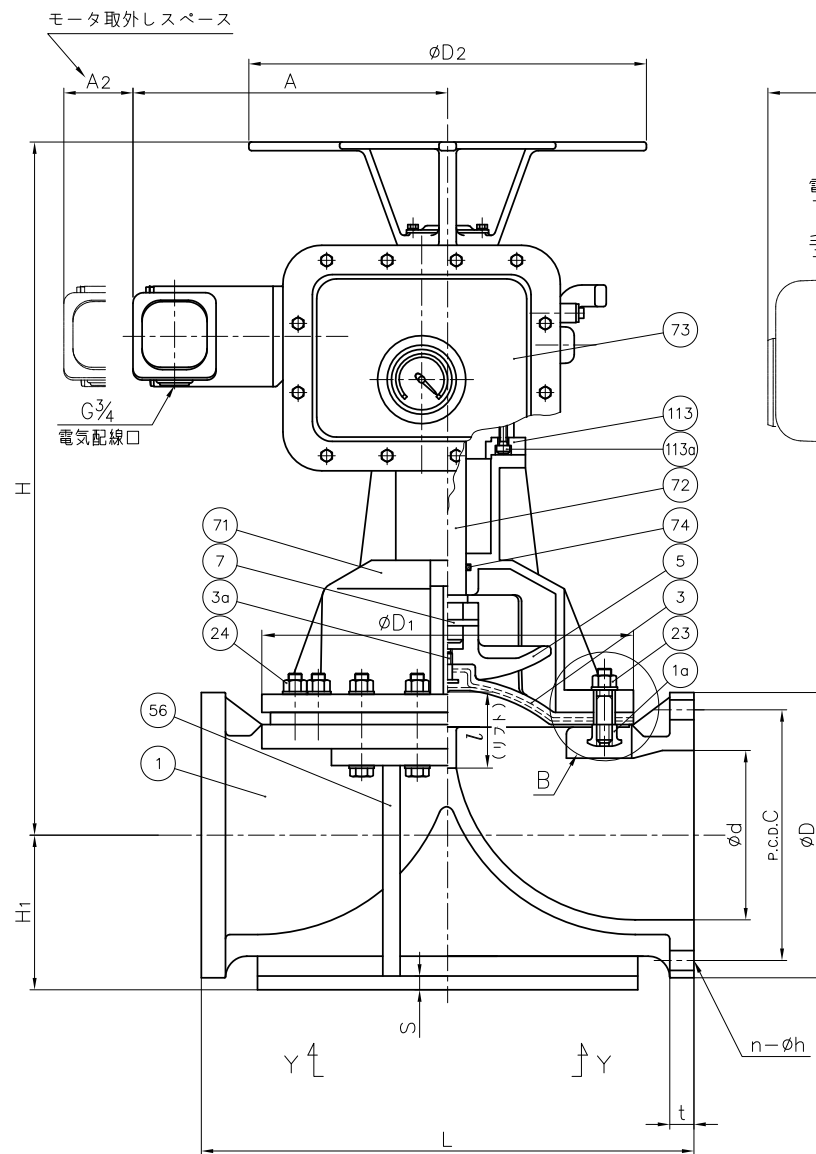
寸法表
