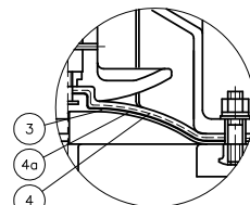
ダイヤフラム材質がPTFEで クッションカバー付の場合
