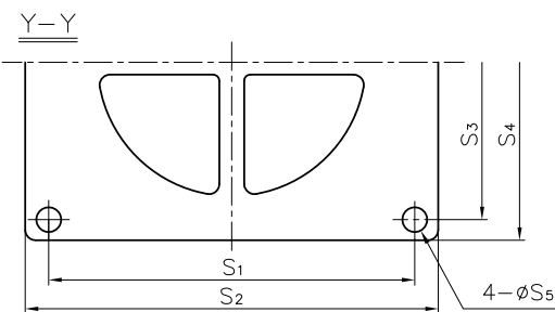
ダイヤフラム材質がPTFEの場合
