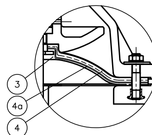
ダイアフラム材質がPTFEで クッションカバー付の場合
