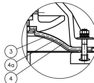
ダイアフラム材質がPTFEで クッションカバー付の場合
