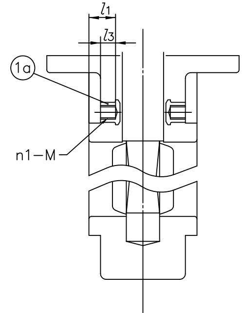
ボディ埋め込み金具詳細
