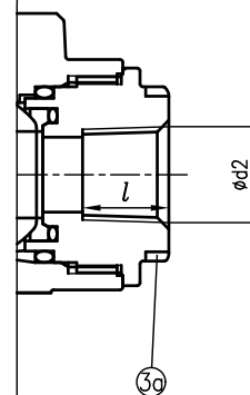
ねじ込み形
