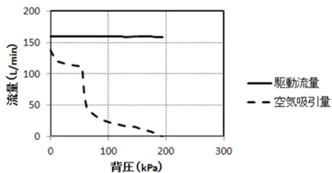
背圧と空気吸引量（呼び径32mm）
