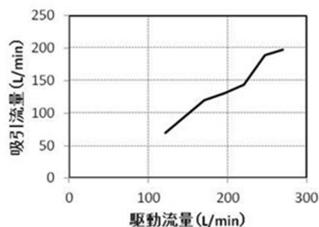
駆動流量と空気吸引量(呼び径40mm)
