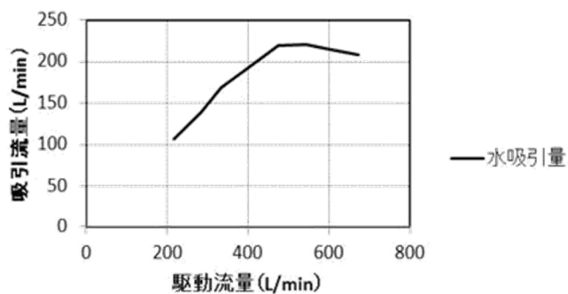
駆動流量と水吸引量(呼び径65mm)
