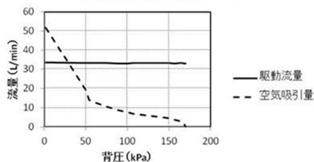
背圧と空気吸引量（呼び径20mm）
