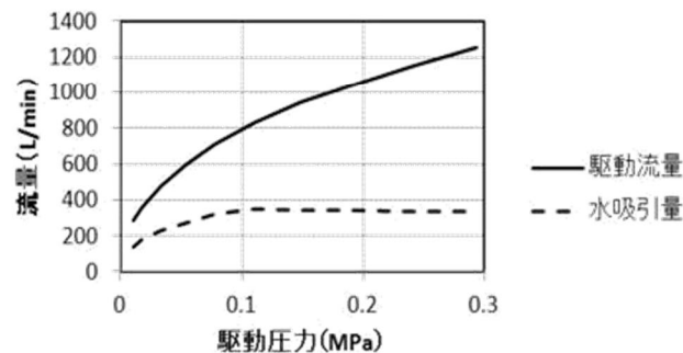
駆動流量と水吸引量(呼び径80mm)
