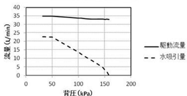
背圧と水吸引量（呼び径20mm）
