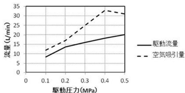
駆動流量と空気吸引量(呼び径15mm)
