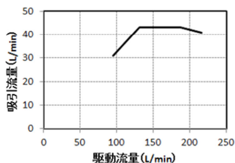
駆動流量と水吸引量(呼び径32mm)
