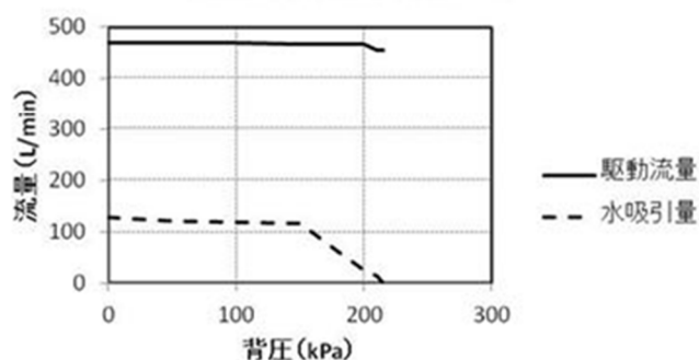
背圧と水吸引量(呼び径50mm)
