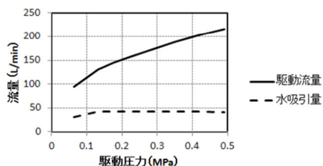
駆動流量と水吸引量(呼び径32mm)
