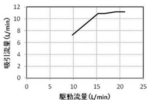
駆動流量と水吸引量(呼び径15mm)
