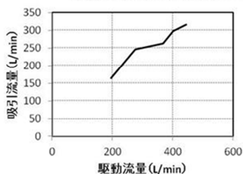
駆動流量と空気吸引量(呼び径50mm)
