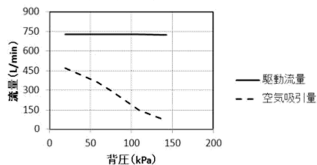
背圧と空気吸引量(呼び径65mm)
