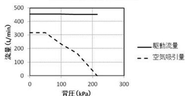
背圧と空気吸引量(呼び径50mm)
