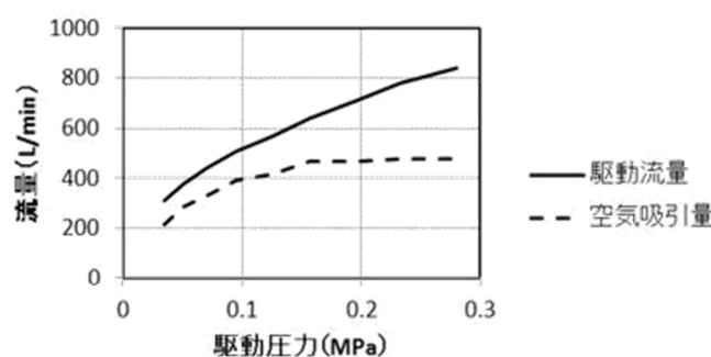
駆動流量と空気吸引量(呼び径65mm)
