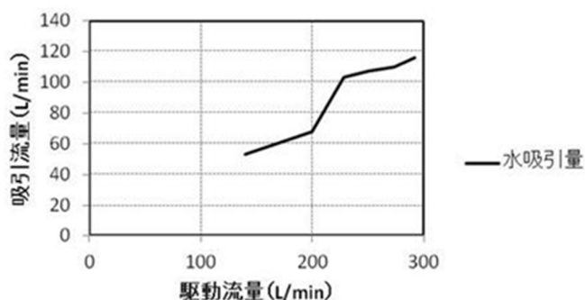
駆動流量と水吸引量(呼び径40mm)
