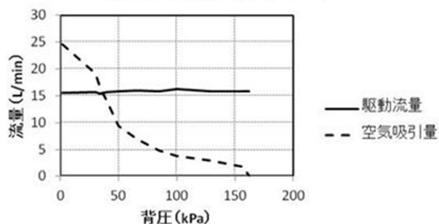
背圧と空気吸引量（呼び径15mm）
