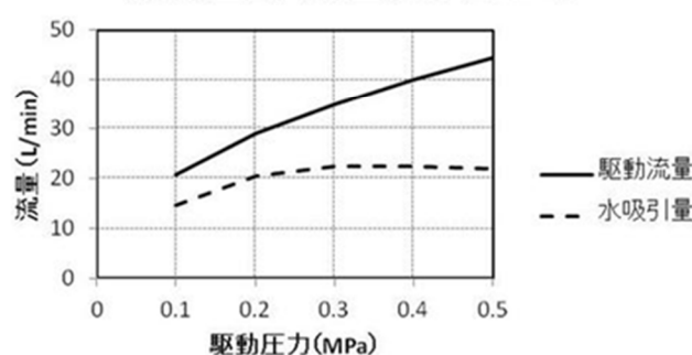
駆動流量と水吸引量(呼び径20mm)
