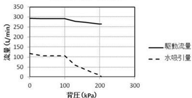
背圧と水吸引量(呼び径40mm)
