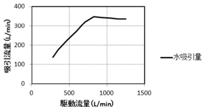
駆動流量と水吸引量(呼び径80mm)
