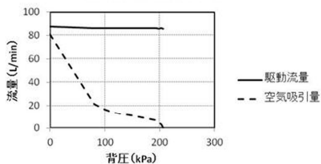
背圧と空気吸引量（呼び径25mm）
