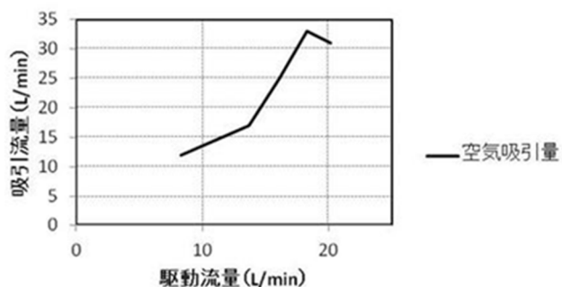
駆動流量と空気吸引量(呼び径15mm)
