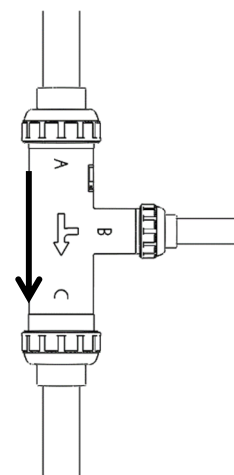
③ 下向き配管 出口側に若干の背圧が必要
