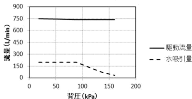
背圧と水吸引量(呼び径65mm)
