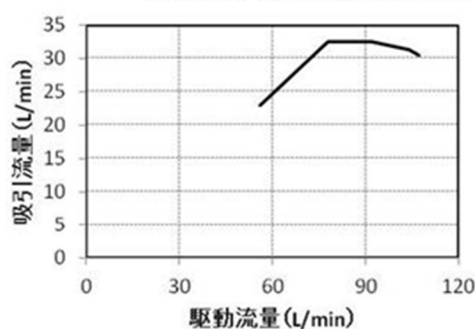
駆動流量と水吸引量(呼び径25mm)
