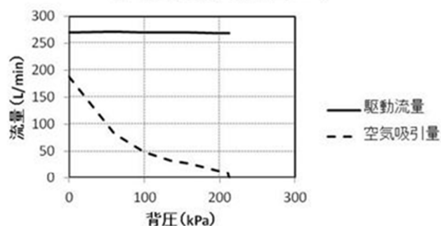
背圧と空気吸引量(呼び径40mm)
