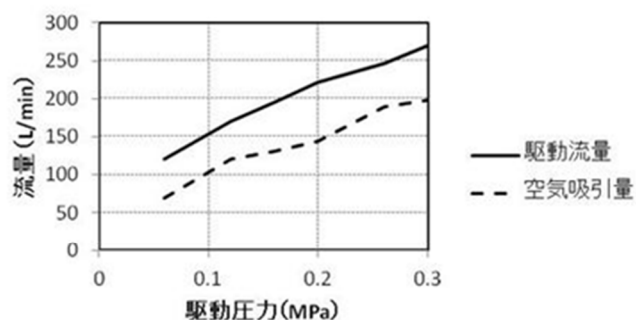
駆動流量と空気吸引量(呼び径40mm)
