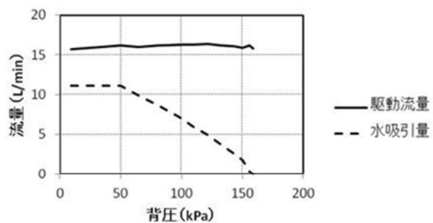
背圧と水吸引量（呼び径15mm）
