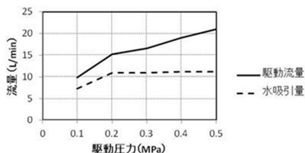
駆動流量と水吸引量(呼び径15mm)
