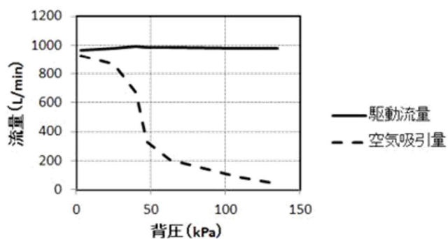
背圧と空気吸引量(呼び径80mm)
