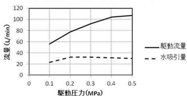
駆動流量と水吸引量(呼び径25mm)
