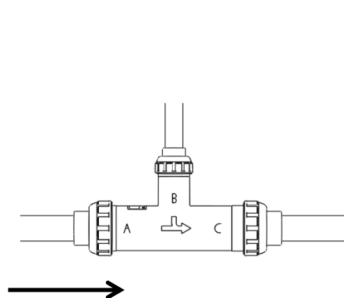
① 水平配管 B ポートの向きは任意
