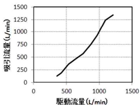
駆動流量と空気吸引量(呼び径80mm)
