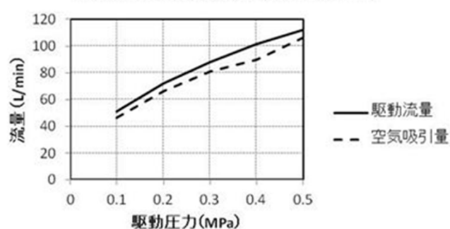
駆動流量と空気吸引量(呼び径25mm)
