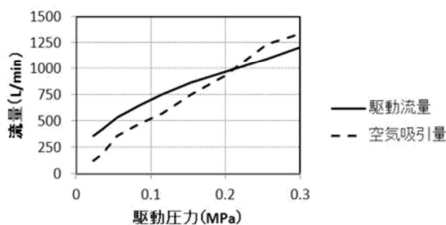
駆動流量と空気吸引量(呼び径80mm)
