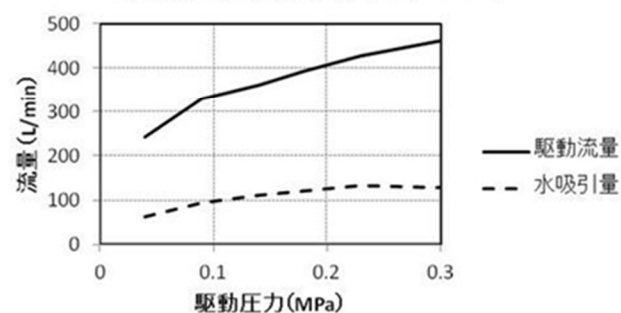
駆動流量と水吸引量(呼び径50mm)
