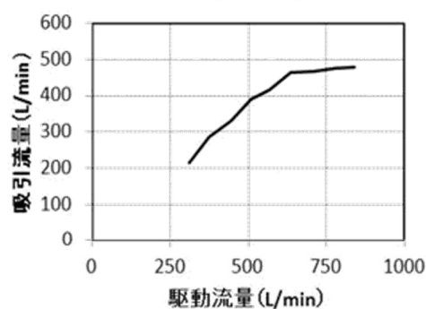
駆動流量と空気吸引量(呼び径65mm)
