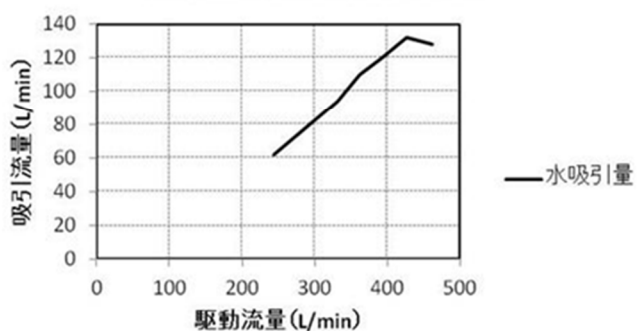
駆動流量と水吸引量(呼び径50mm)
