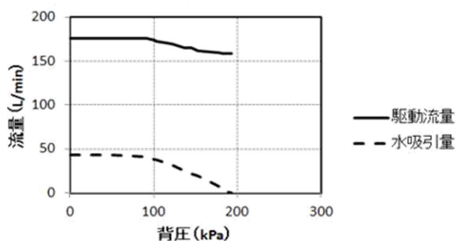
背圧と水吸引量（呼び径32mm）
