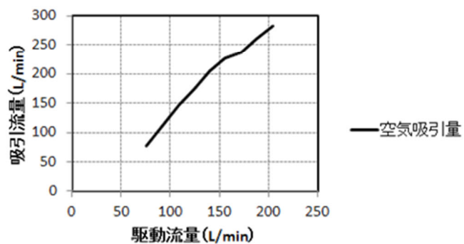
駆動流量と空気吸引量(呼び径32mm)
