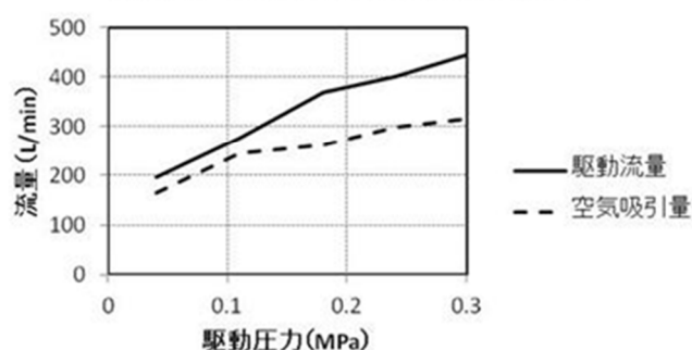
駆動流量と空気吸引量(呼び径50mm)
