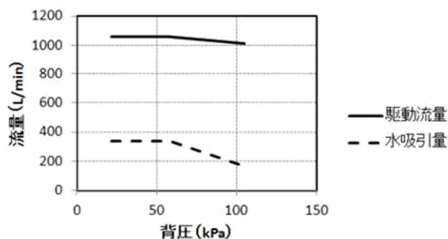
背圧と水吸引量(呼び径80mm)
