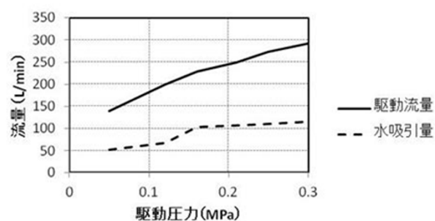
駆動流量と水吸引量(呼び径40mm)
