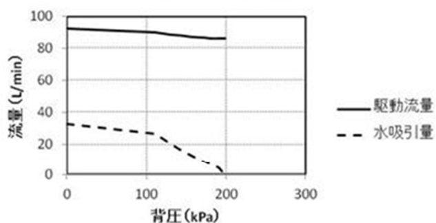
背圧と水吸引量（呼び径25mm）
