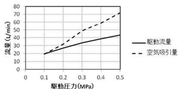
駆動流量と空気吸引量(呼び径20mm)
