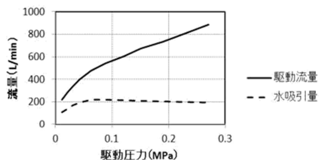
駆動流量と水吸引量(呼び径65mm)
