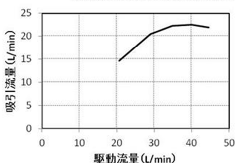
駆動流量と水吸引量(呼び径20mm)
