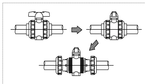
ボールバルブ 21 型
