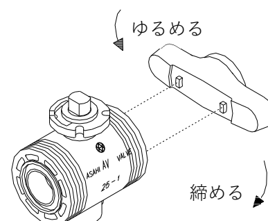
ボールバルブ 21α 型
