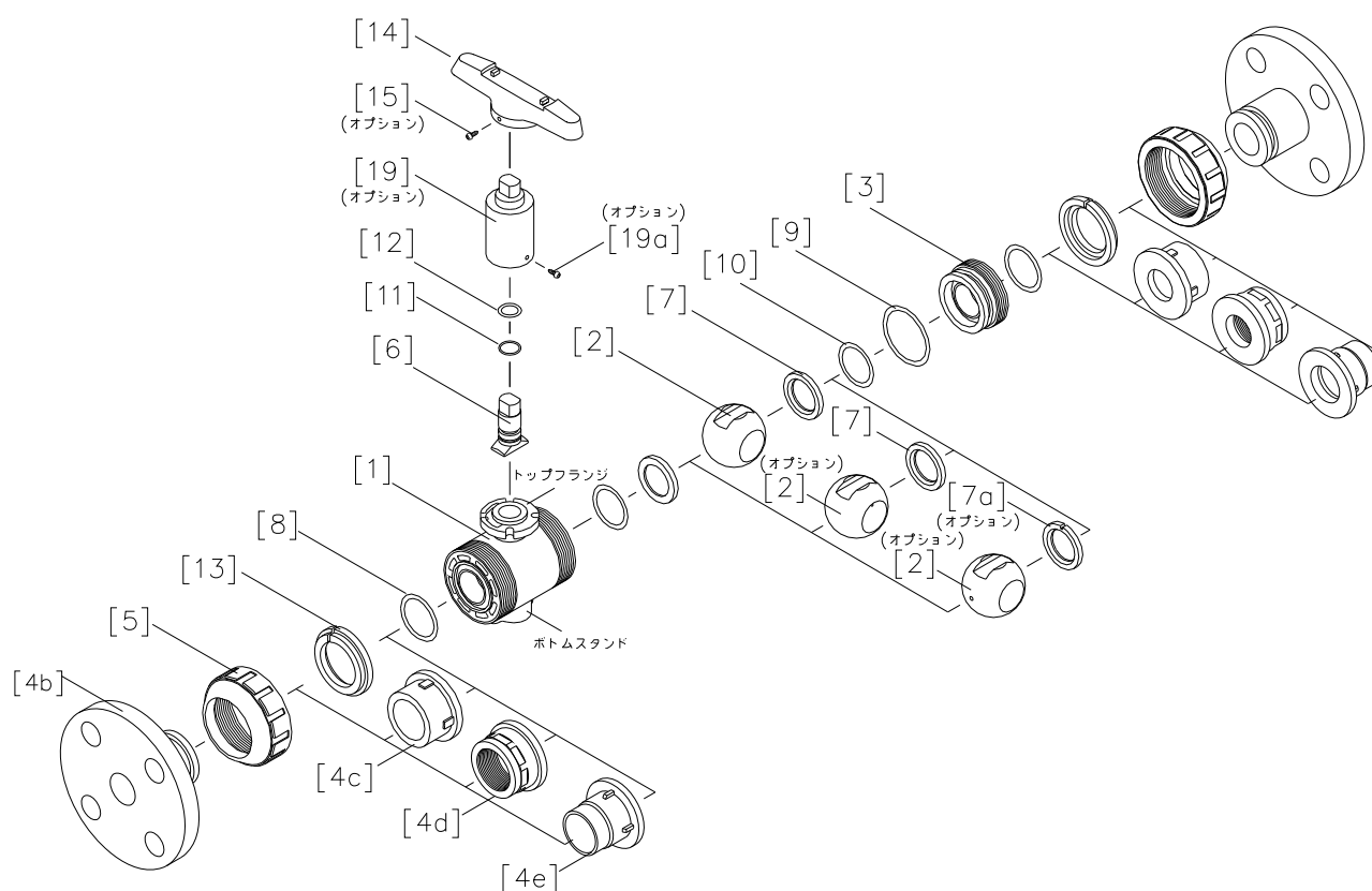
バルブ部品表
