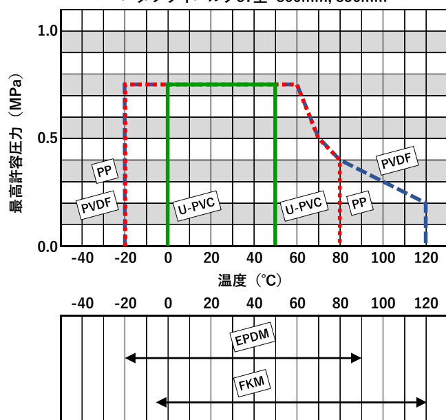
バタフライバルブ57型 300mm, 350mm
