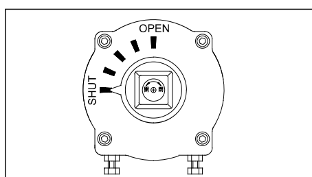
全閉状態
