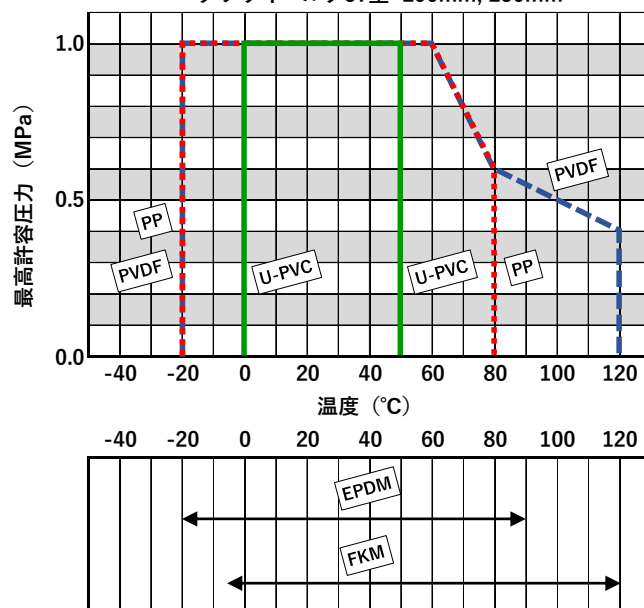
バタフライバルブ57型 200mm, 250mm
