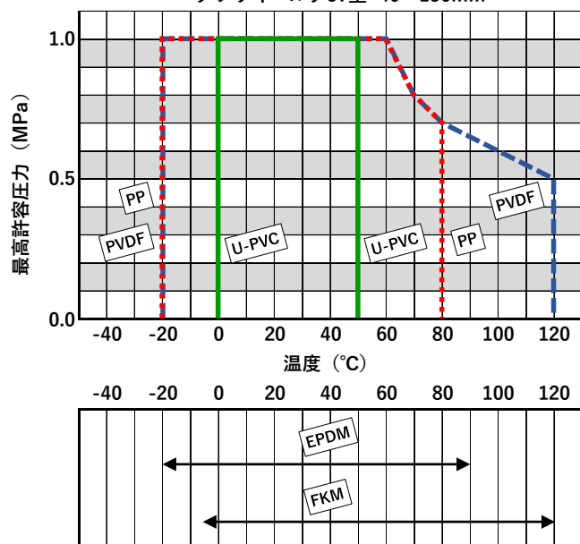
バタフライバルブ57型 40～150mm
