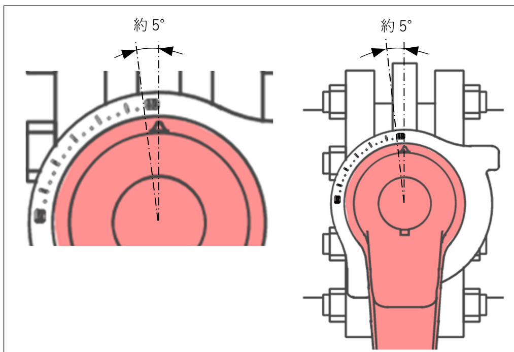
図 6-1 全閉状態（拡大図）
