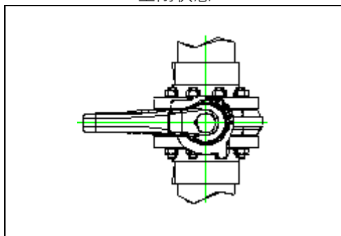
全閉状態
