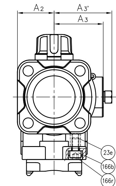
フランジ形
