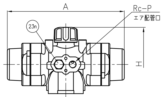
アクチュエータ形状（AR040）
