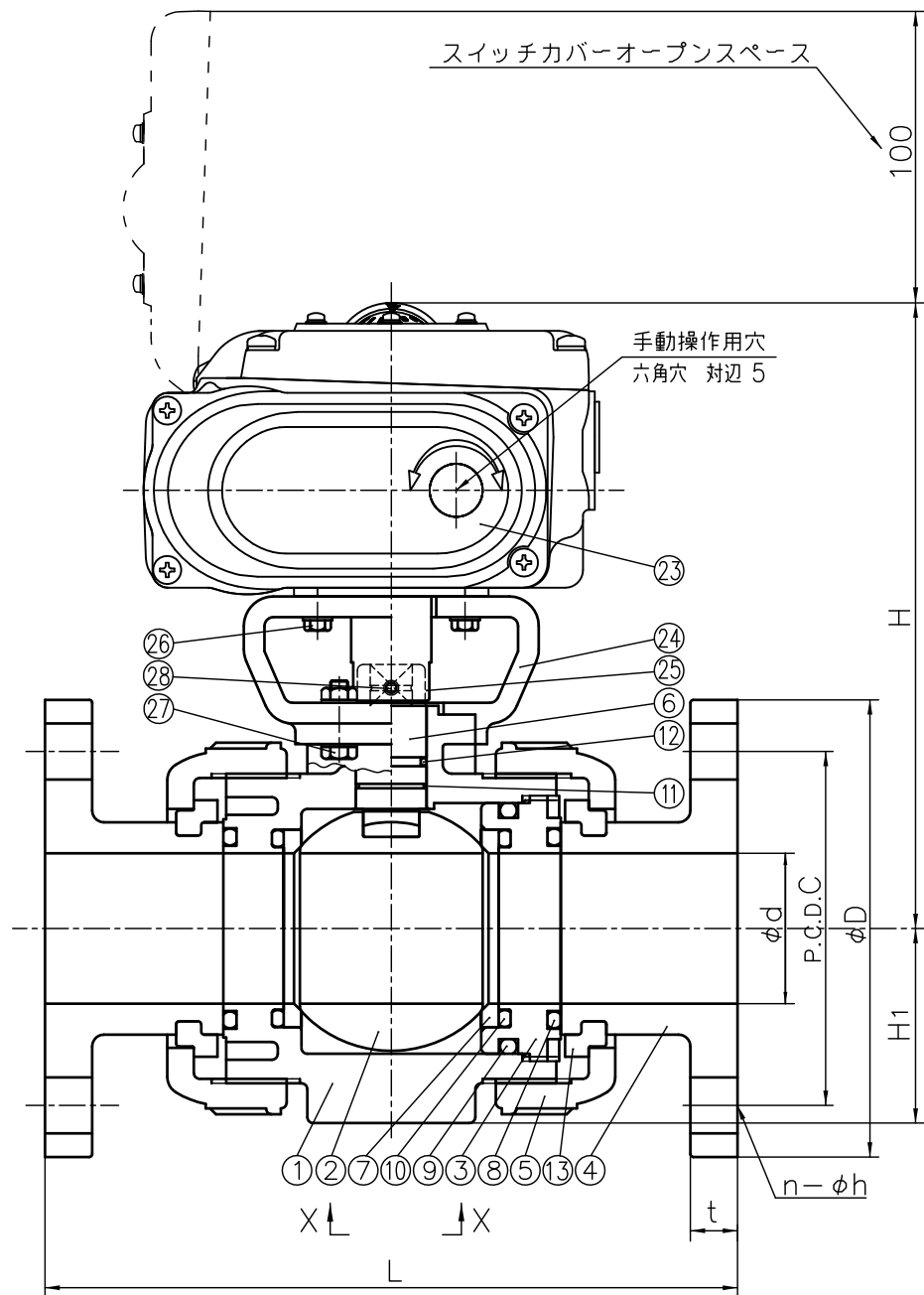
フランジ形
