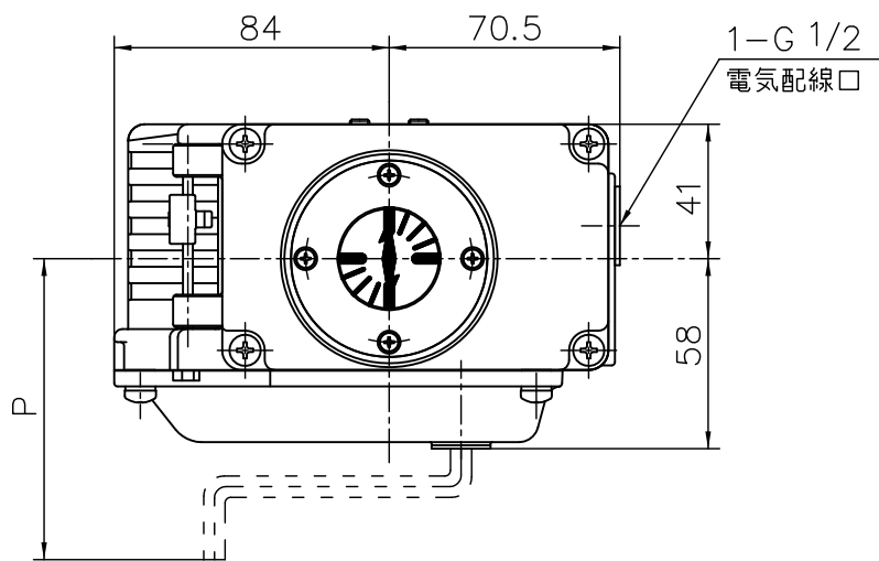
フランジ形
