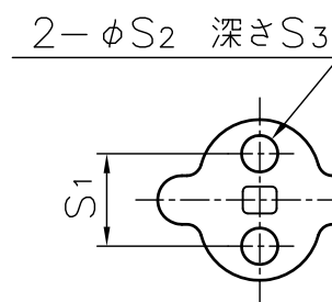
インザート金具取付穴部詳細
