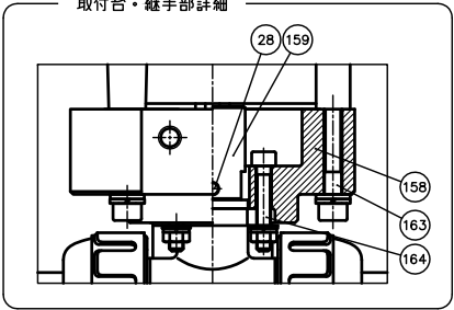
取付台・継手部詳細
