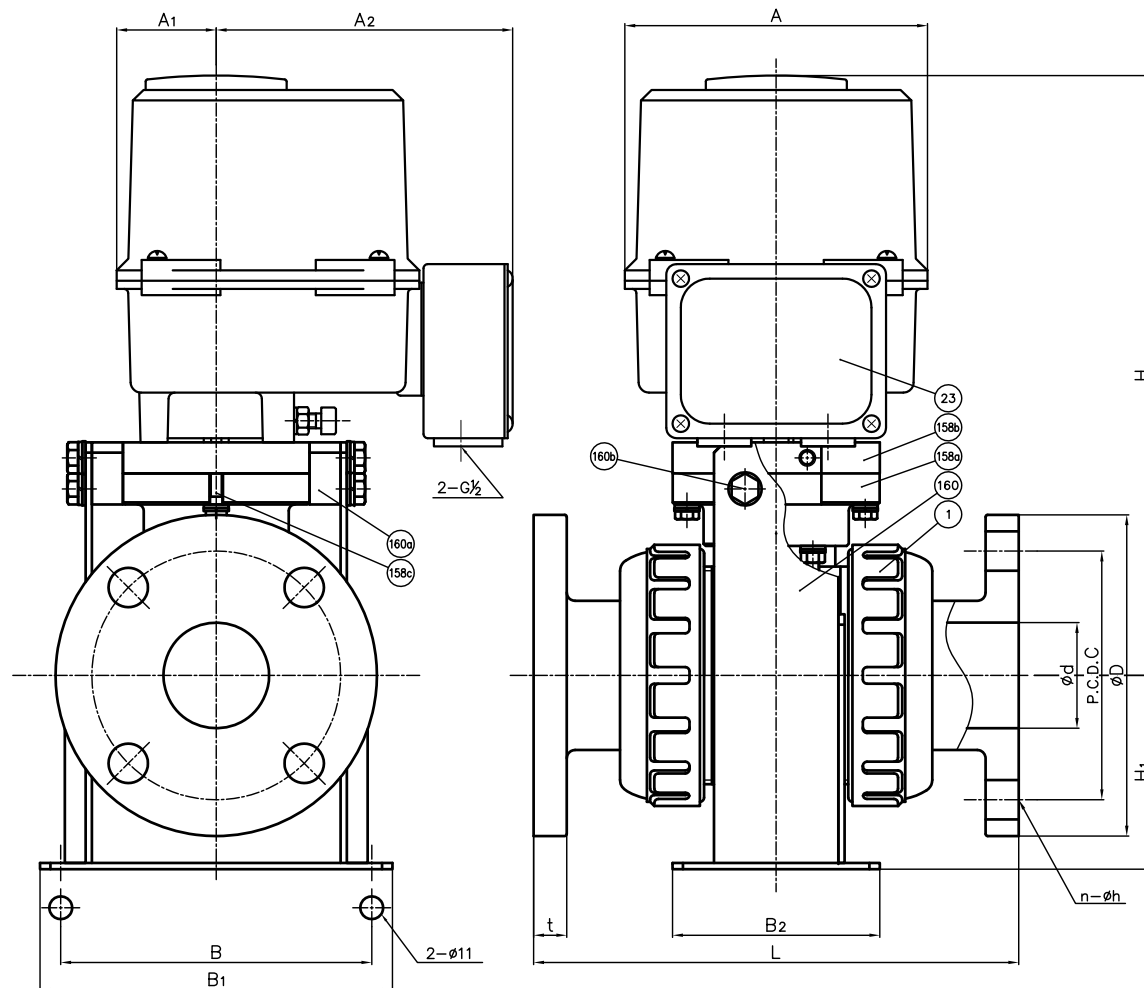
フランジ形
