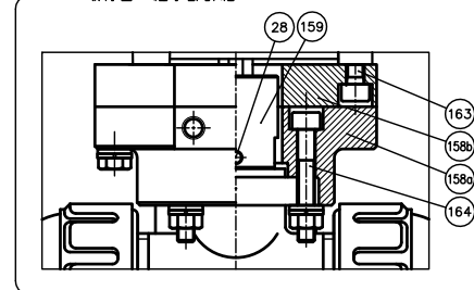
取付台・継手部詳細
