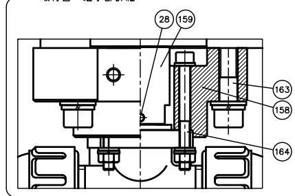
取付台・継手部詳細
