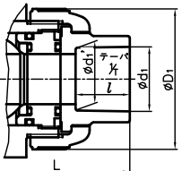
ソケット形
