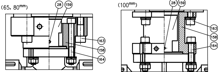
取付台・継手部詳細
