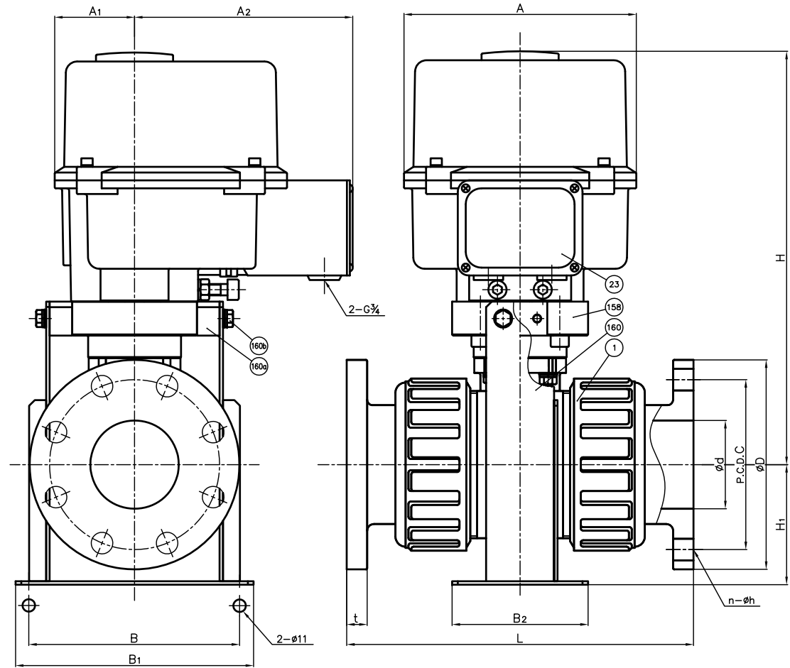
フランジ形
