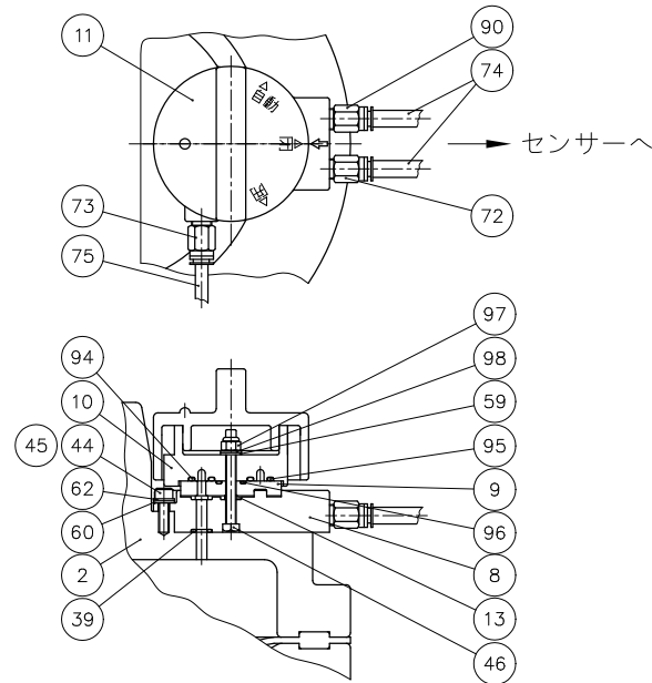
ポンネット上部 切り換えバルブ詳細図
