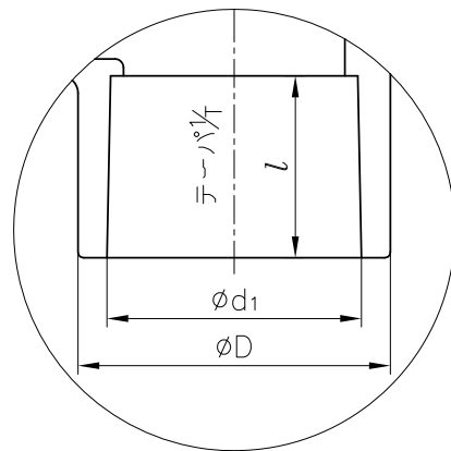
ソケット形の場合
