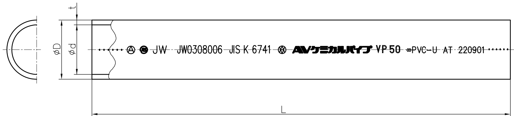
寸法表
