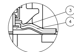
ダイヤフラムがPTFEの場合
