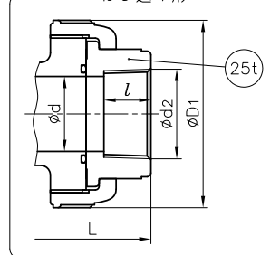
ねじ込み形
