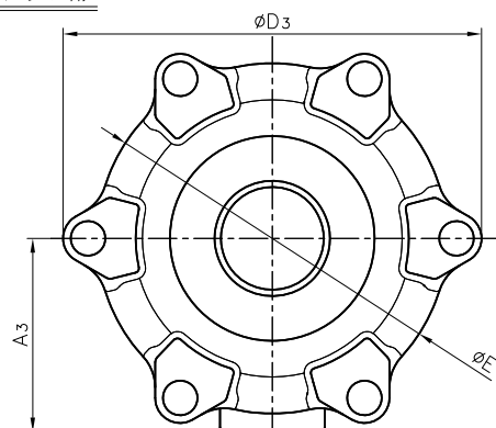
ソケット形
