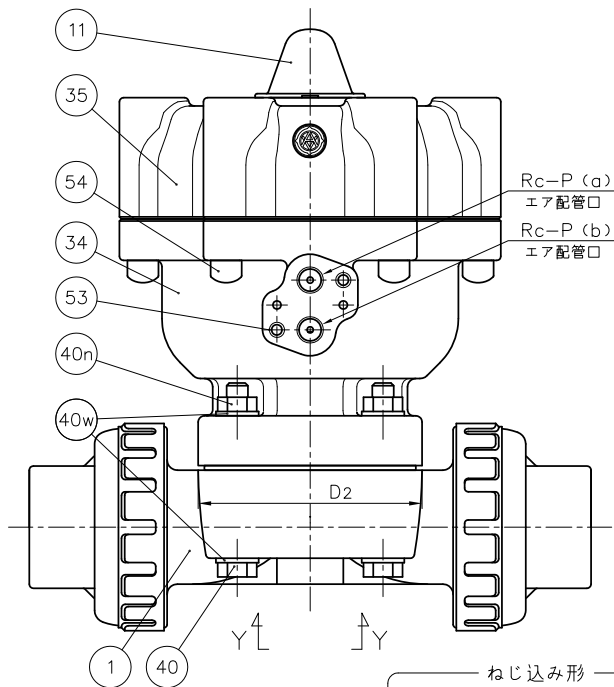
ねじ込み形
