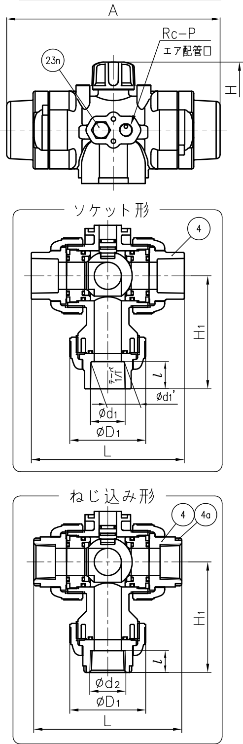
アクチュエータ形状 (AR040)
