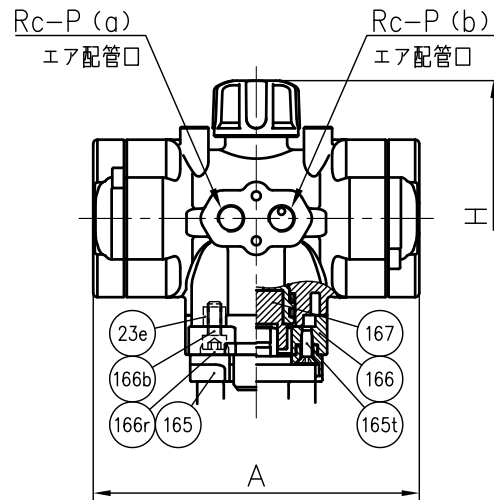
アクチュエータ形状 (AR040)
