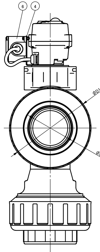
端子番号と流路の関係
