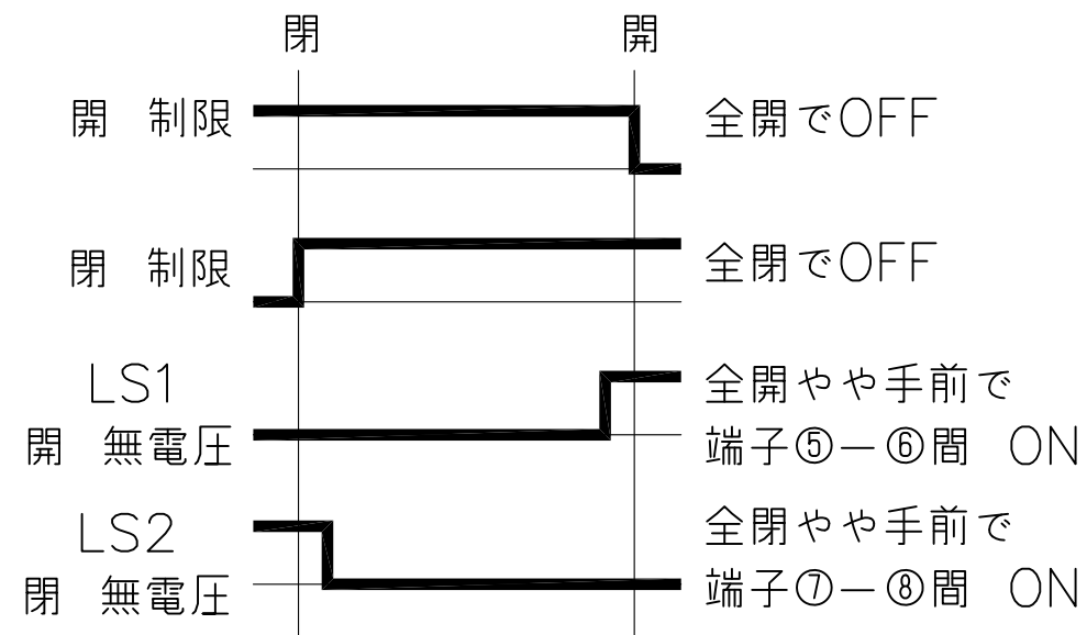
緊急遮断弁のスイッチングチャート
