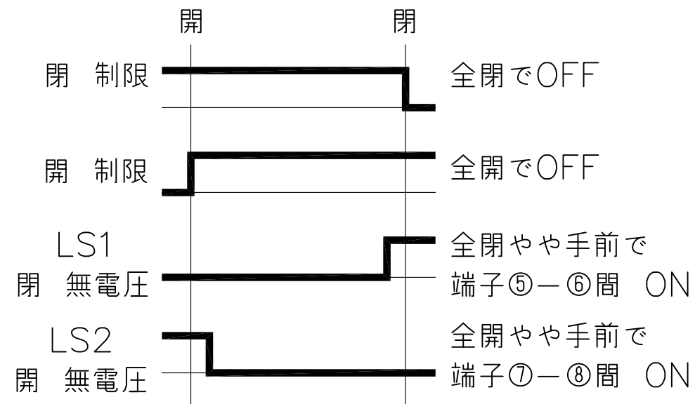
緊急開放弁のスイッチングチャート
