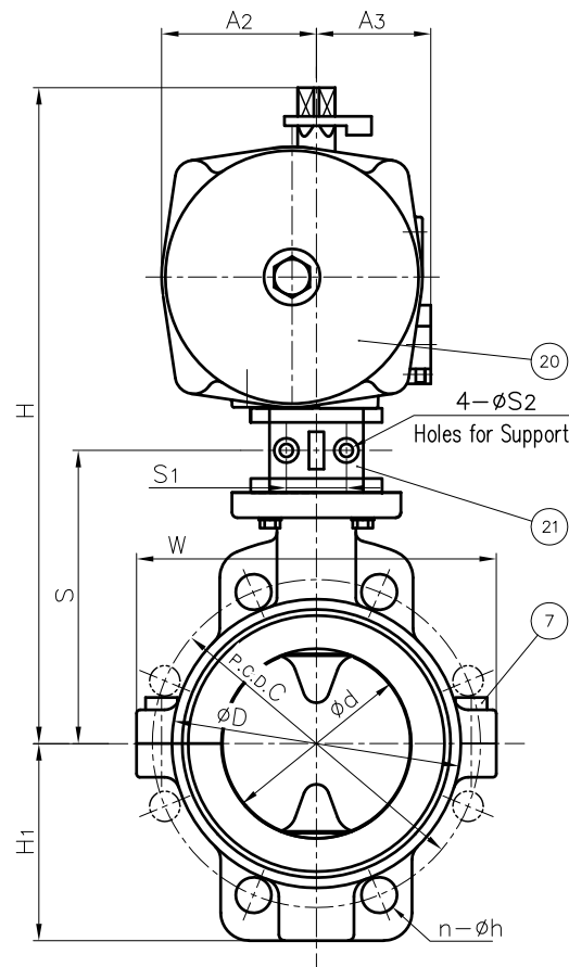
DIMENSIONS TABLE
