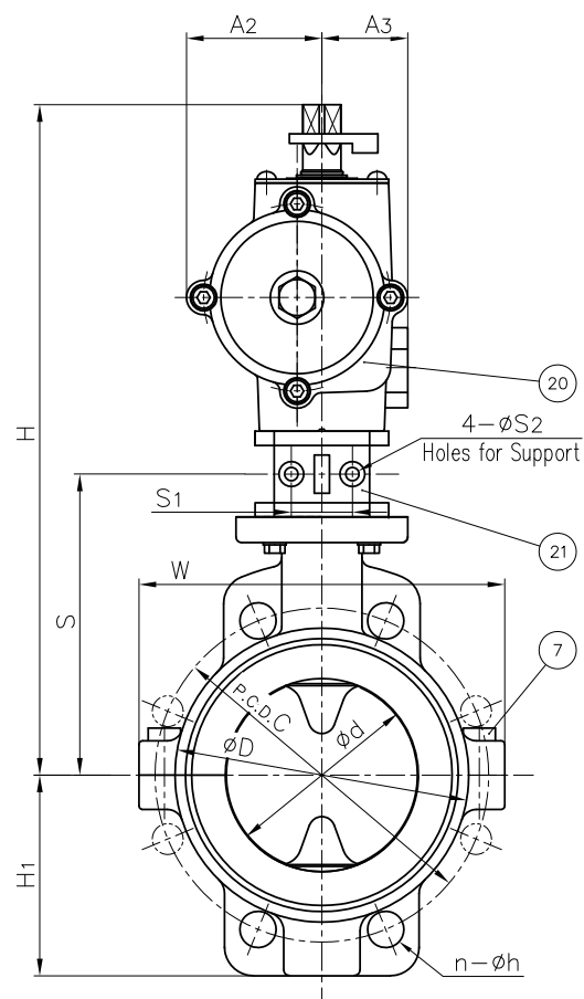
DIMENSIONS TABLE
