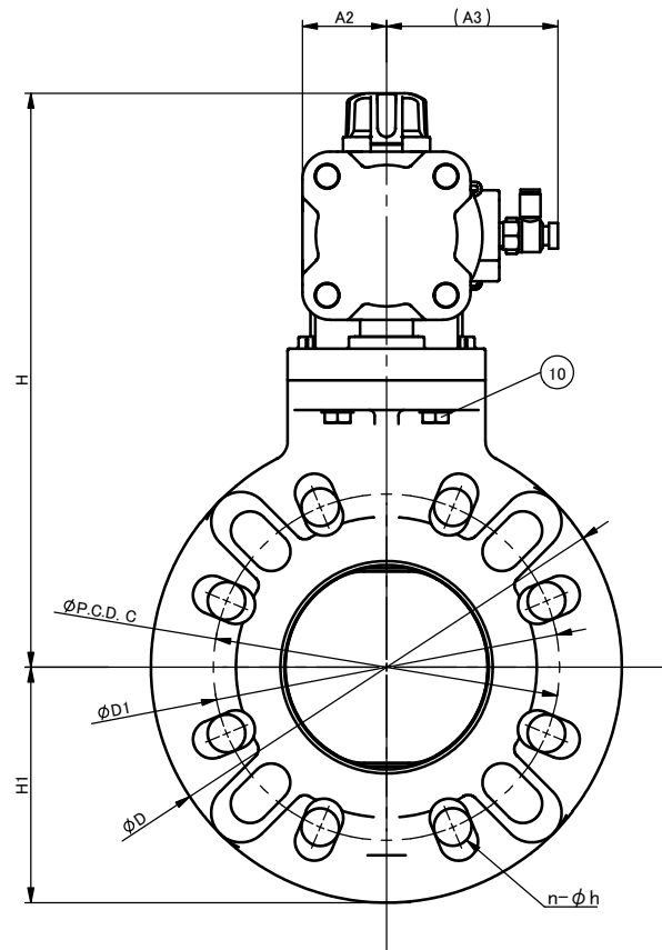
DIMENSIONS TABLE
